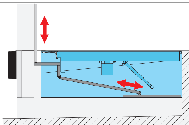
schéma général 5145.0140
